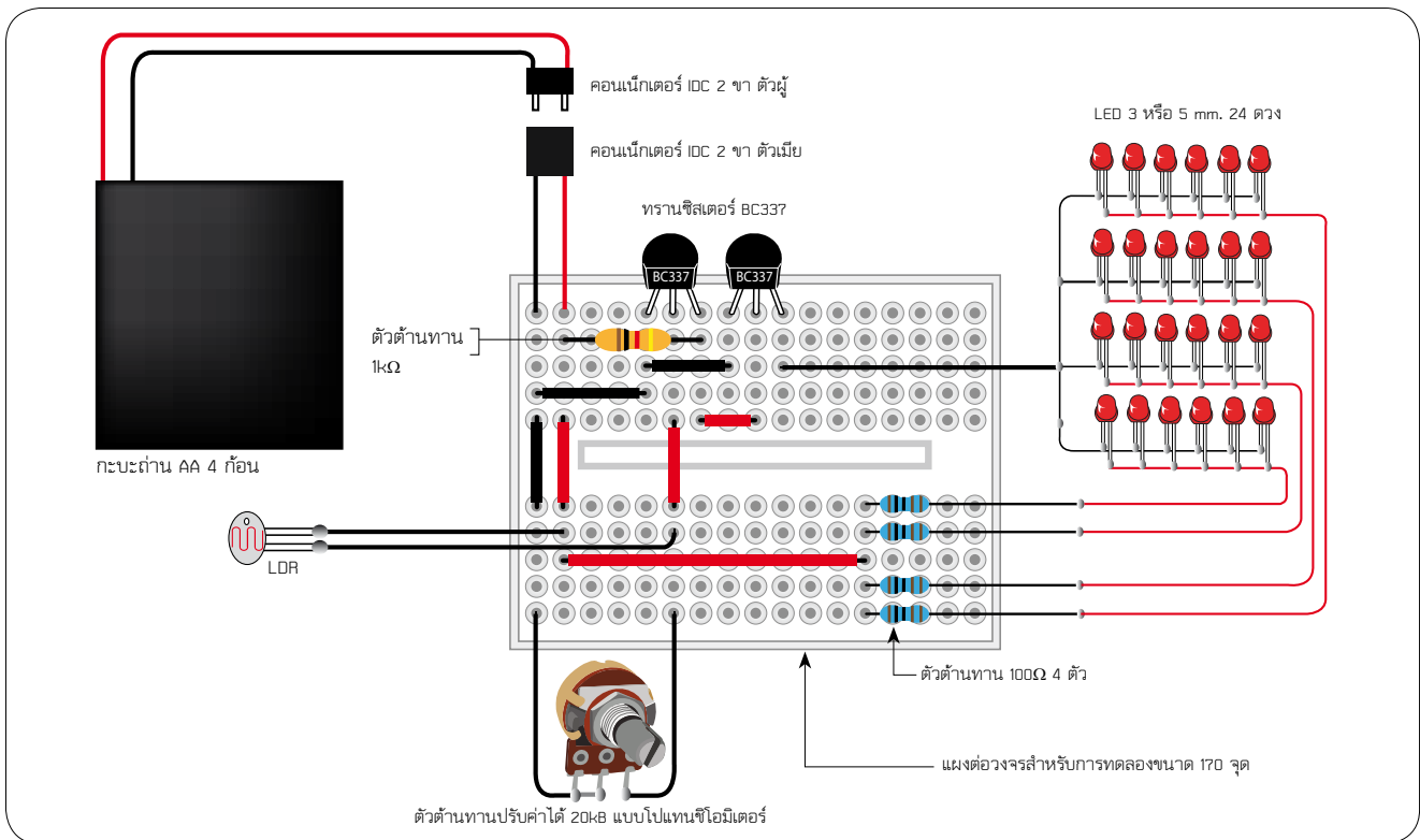
รูปแสดงการเชื่อมต่อวงจรของโครงการ Flower lamp
